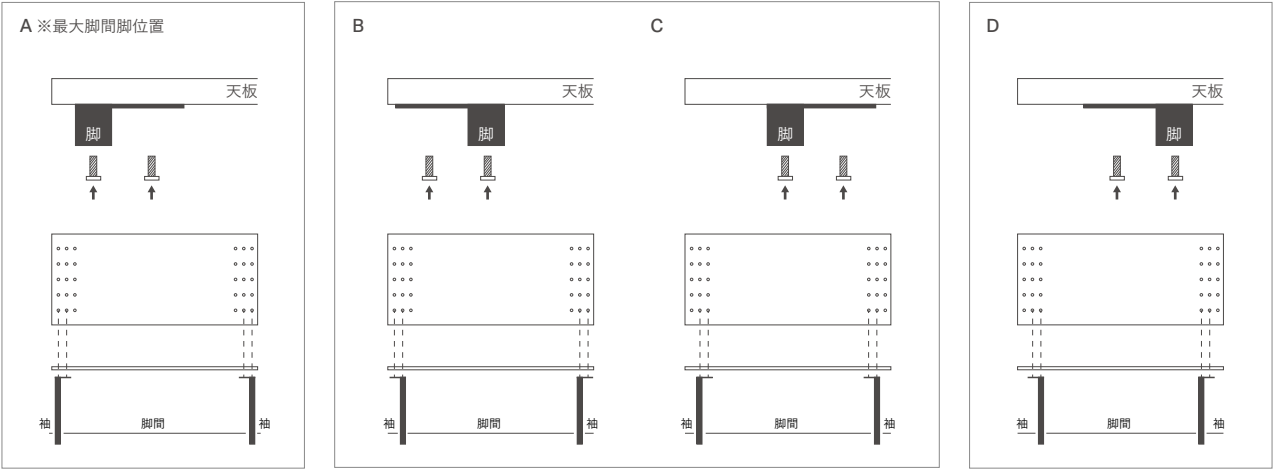
脚位置パターン A-D
